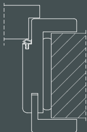
Esecuzione Standard, pannello con battuta
