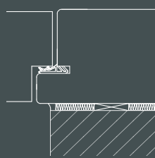
Telaio BR 68, doppia battuta
