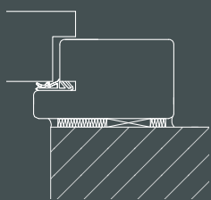
Telaio BR 45, pannello con battuta
