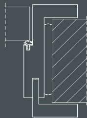
Esecuzione a spigolo vivo, pannello a filo telaio
