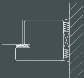
Telaio BR 68, pannello a filo telaio
