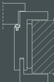
Esecuzione a spigolo vivo, pannello con battuta
