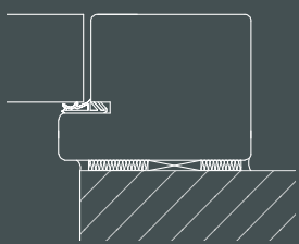
Telaio BR 68, pannello a filo telaio
