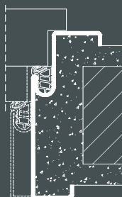
Telaio in ferro, pannello con battuta
