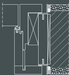
telaio speciale per pannello a filo telaio
