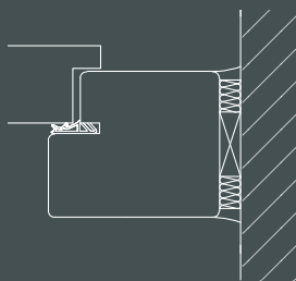
Telaio BR 68, pannello con battuta
