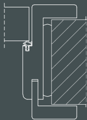
Esecuzione Standard, pannello a filo telaio
