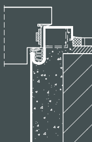
Telaio in ferro, pannello con battuta, E130 VKF, Valore fonico R_w=47 dB (valore per pannello)
