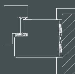
Telaio BE 68, doppia battuta
