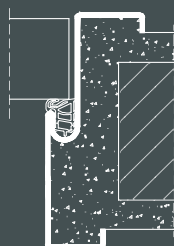
Telaio in ferro, pannello a filo telaio
